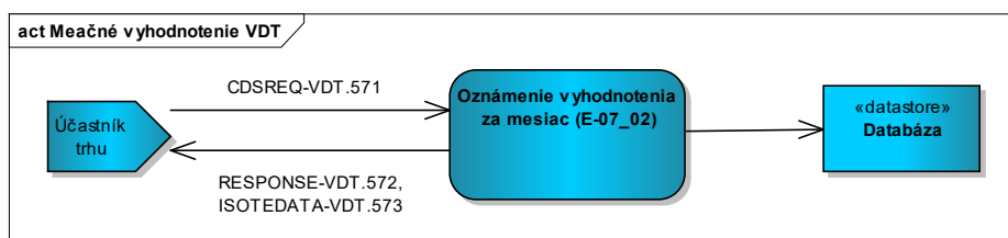
Obrázok 37 Obrázok 38 Schéma oznámenia vyhodnotenia VDT za mesiac pre ÚT
