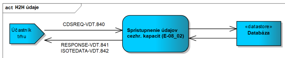
Obrázok 28 Obrázok 29 Schéma príjmu údajov cezhr. kapacít
