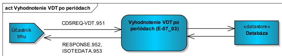
Obrázok 38 Obrázok 39 Schéma oznámenia vyhodnotenia VDT po periódach pre ÚT
