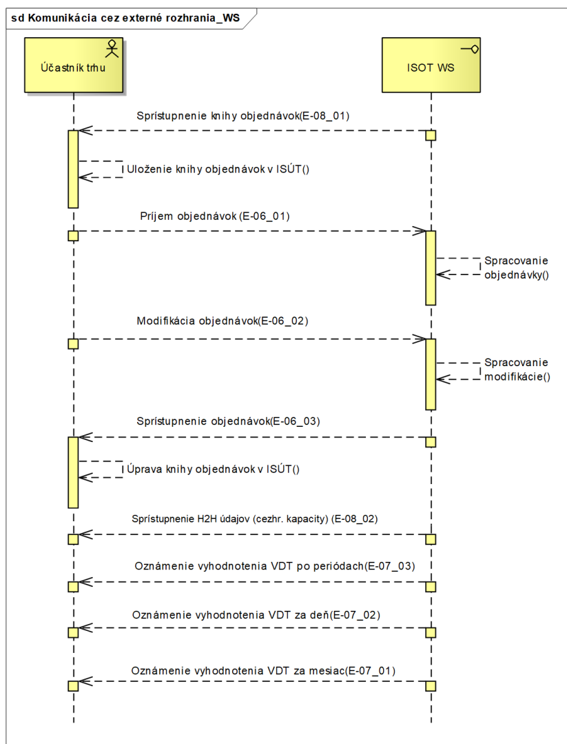
Obrázok 5 Komunikačný scenár webových služieb v režime koordinovaného organizovania vnútrodnenného trhu
