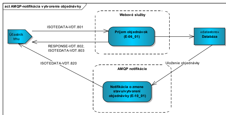
Obrázok 39 Obrázok 40 Schéma posielaných správ – vytvorenie objednávky (AMQP notifikácia)
