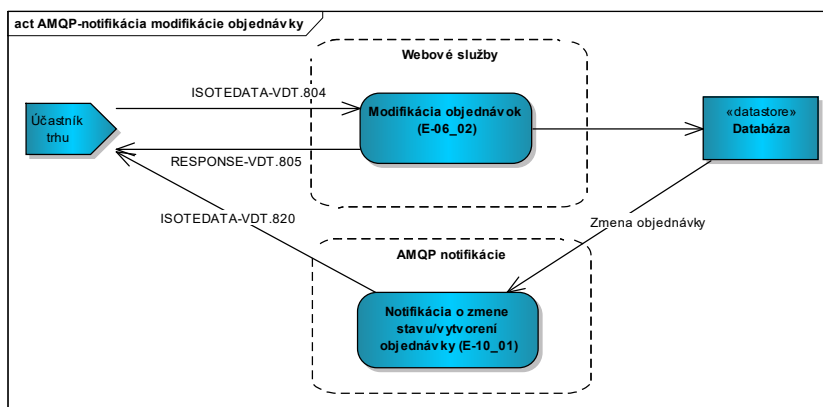
Obrázok 41 Obrázok 42 Schéma posielaných správ – modifikácia objednávky (AMQP notifikácia)
