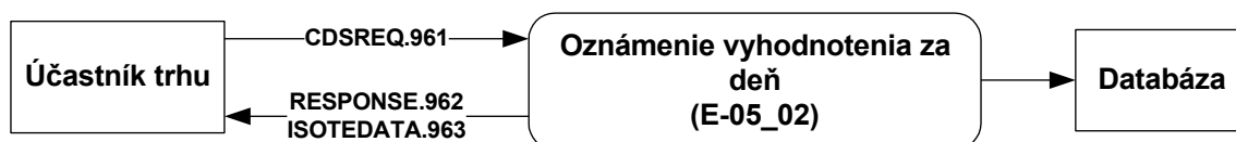
Obrázok 35 Obrázok 36 Schéma oznámenia vyhodnotení DT za deň pre ÚT
