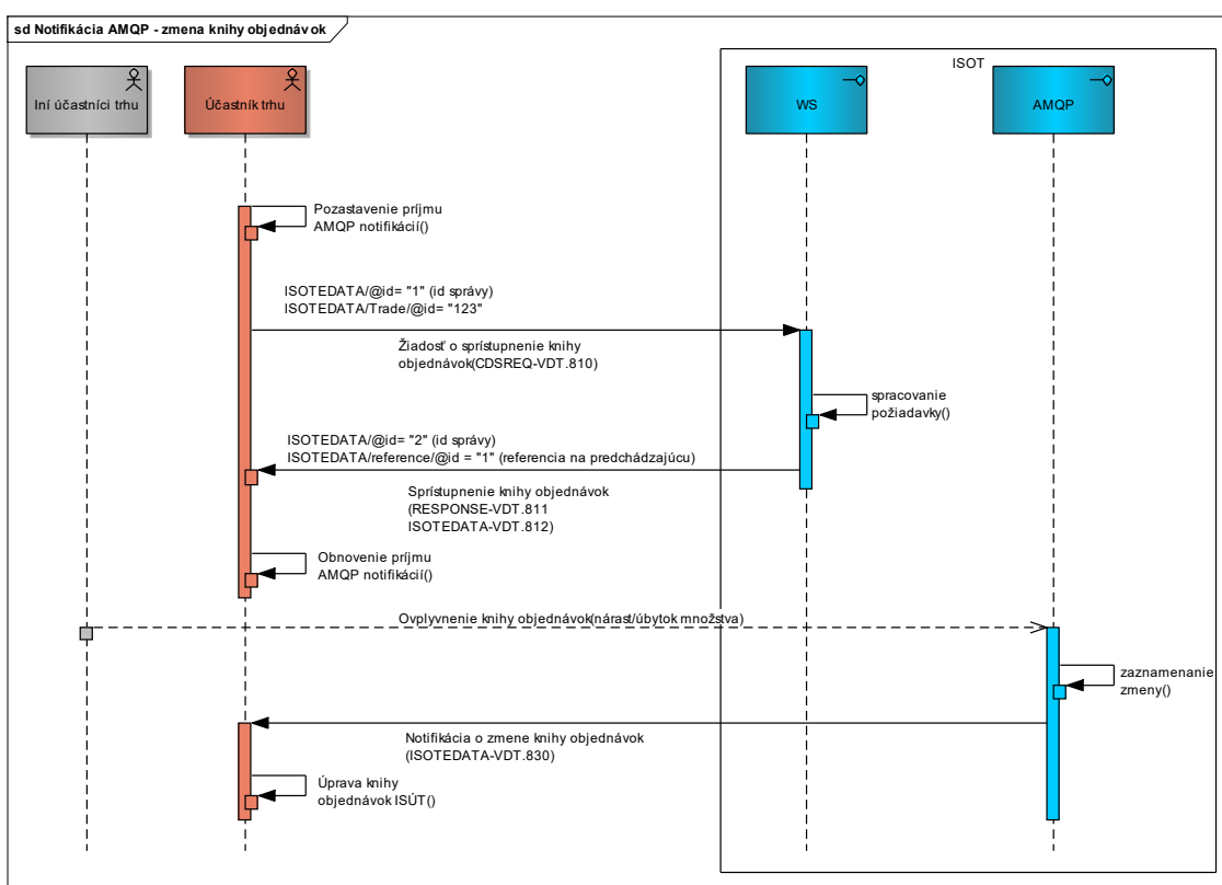
Obrázok 44 Obrázok 45 Schéma následnosti posielaných správ – zmena knihy objednávok (AMQP notifikácia)
