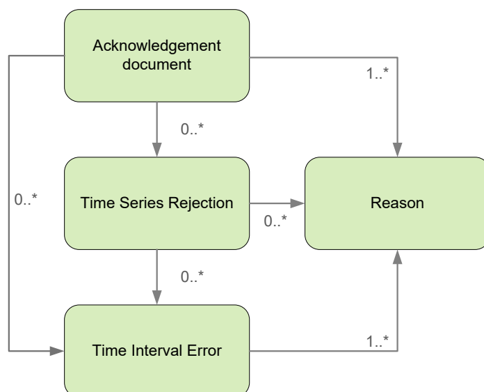
Obrázok 49 Obrázok 50 Schéma štruktúry Acknowledgement
