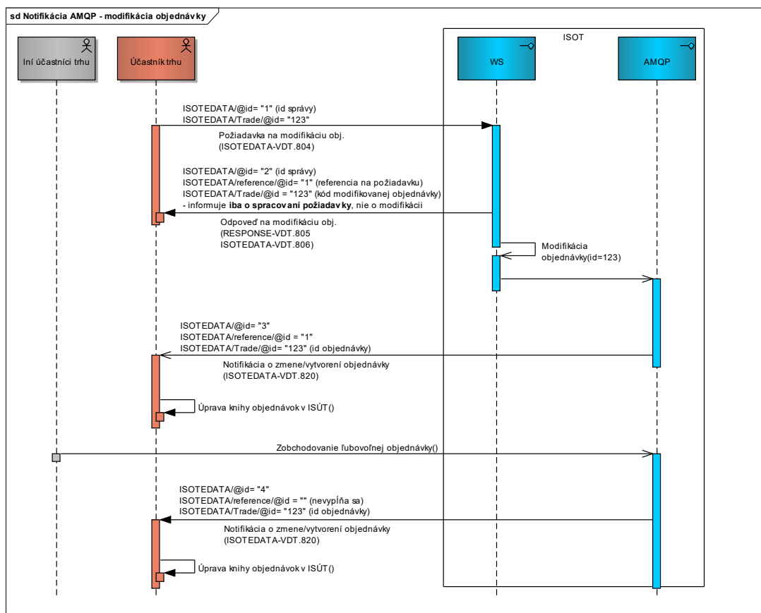
Obrázok 42 Obrázok 43 Schéma následnosti posielaných správ – modifikácia objednávky (AMQP notifikácia)
