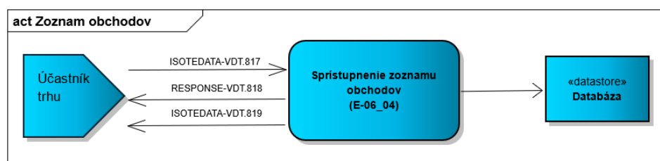
Obrázok 27 Schéma sprístupnenia zoznamu obchodov UT
