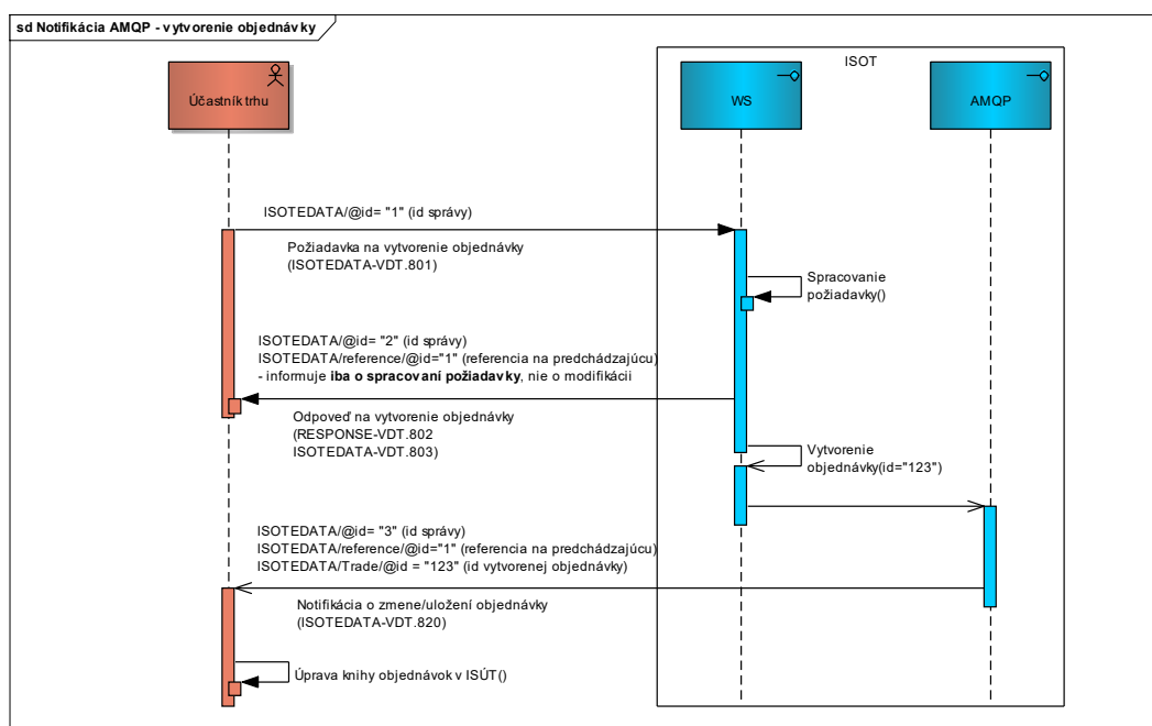
Obrázok 40 Obrázok 41 Schéma následnosti posielaných správ – vytvorenie objednávky (AMQP notifikácia)
