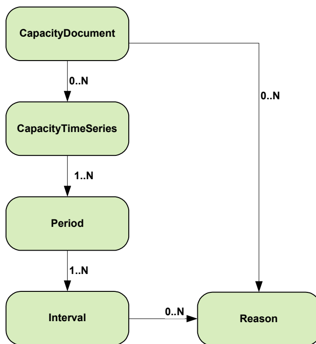
Obrázok 50 Obrázok 51 Schéma štruktúry CapacityDocument
