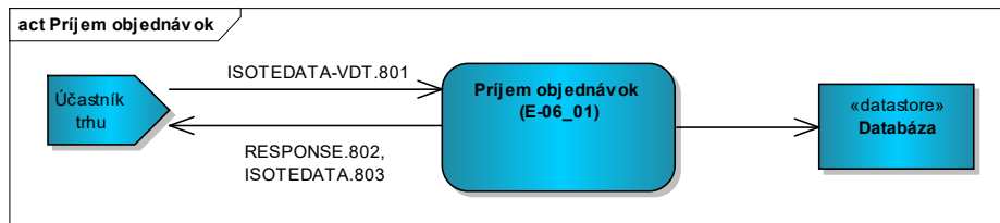
Obrázok 24 Schéma prijmu objednávky ÚT
